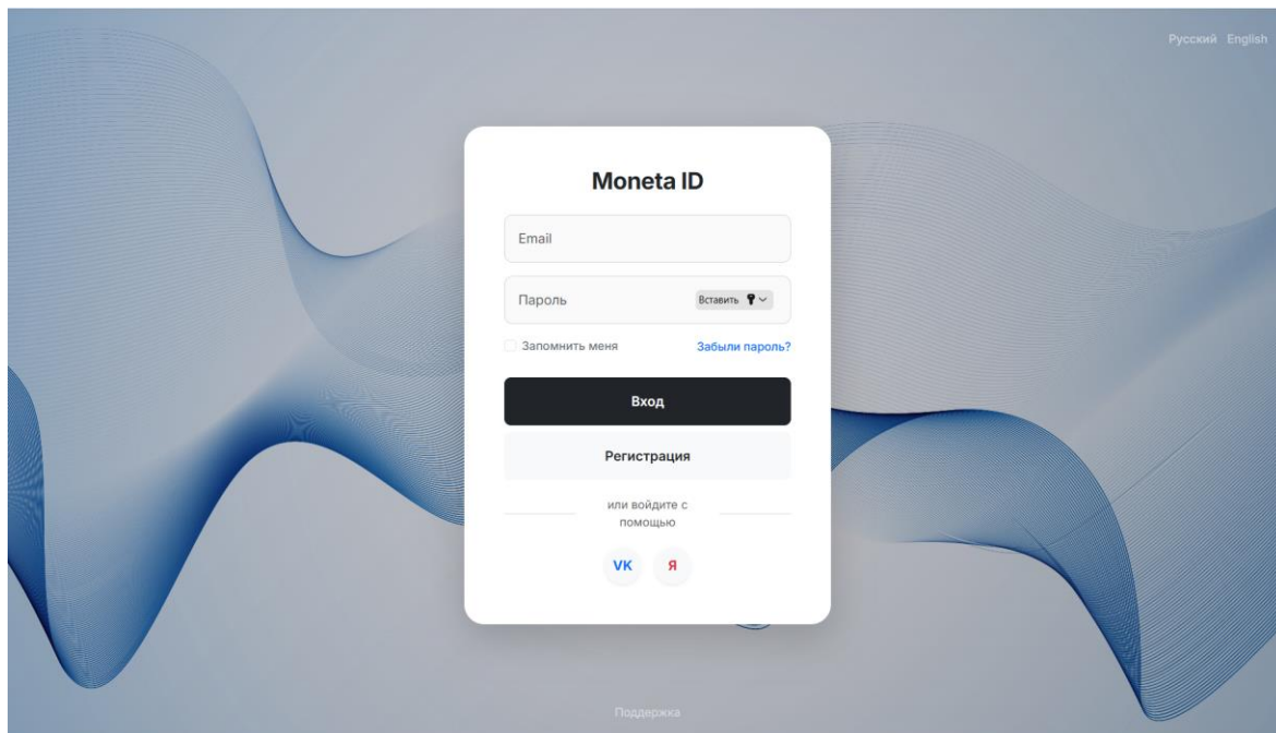
Страница «Вход»
