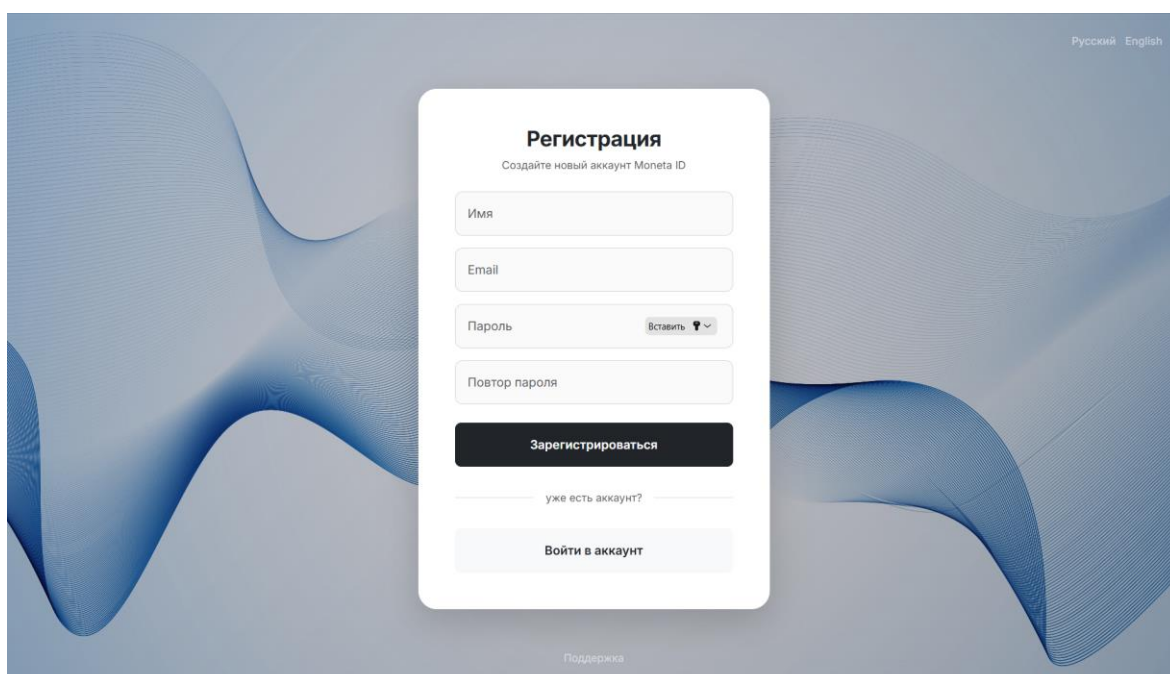
Страница «Регистрация»
