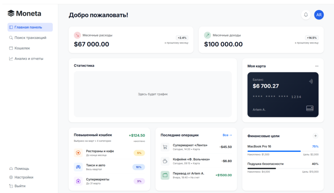
Страница «Дашборд»
